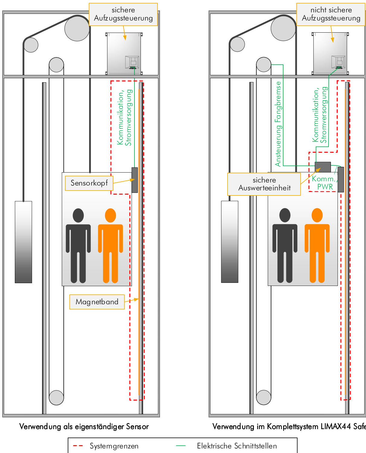
Abbildung 1: LIMAX44 RED als ungeführte Variante zusammen mit einer sicheren Steuerung (links) oder im Verbund mit der sicheren Auswerteeinheit Safe Box als Gesamtsystem LIMAX44 Safe (rechts)
